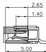
SECTION A-A SCALE 1:1
